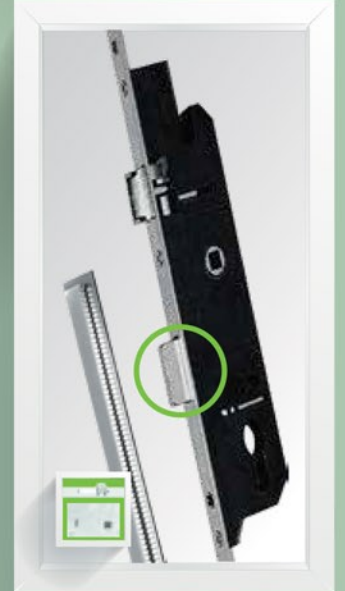
Plastik Gövde Kilitli Kapi İspanyoleti Kesilebilir - Silindirli - Dilli 01.KKİ062.00.00 - 1900 mm (1700-2200 mm)
