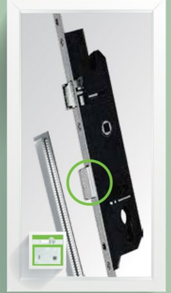
Plastik Gövde Kilitli Kapi İspanyoleti Kesilebilir - Silindirli - Dilli 01.KKİ056.00.00 - 1900 mm (1700-2200 mm)
