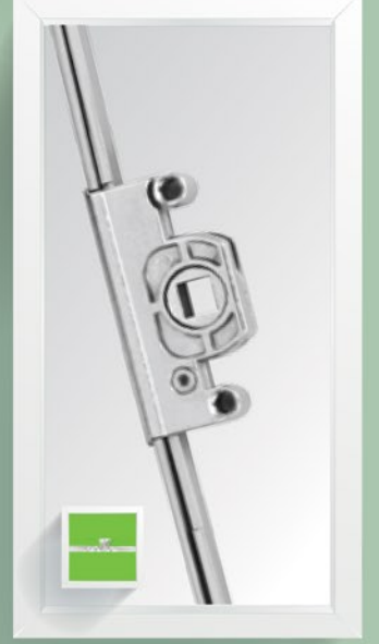
01.TAI201.01.00 - 01.TAI201.10.00 Zamak Gövde Tek Açılım İspanyolet Güvenlik Pimli Boylar: 30, 40, 60, 80, 100, 120, 140, 160, 180, 200 cm
